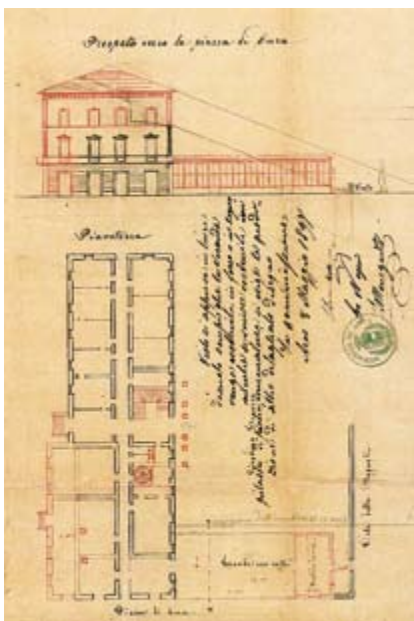
Sopra un prospetto relativo a Casa Strasser verso Piazza di Cura, sotto quello relativo al suo ampliamento.
